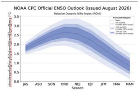
အီကွေတာအနီးရှိ အပူပိုင်းပတ်ဝန်းကျင်သမုဒ္ဒရာ၏ ပင်လယ်ရေမျက်နှာပြင် အပူချိန်ခန့်မှန်းချက်ပြပုံ။
