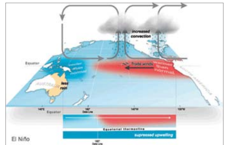
အယ်လ်နီညိုဖြစ်စဉ်များတွင် ပတ်ဝန်းကျင်သမုဒ္ဒရာနှင့် ဆက်စပ်နေသည့် လေထုအခြေအနေပြပုံ။
